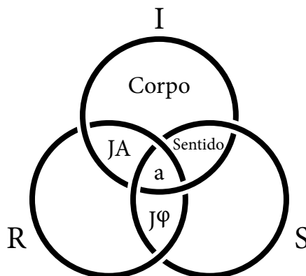
Figura 1. Nó borromeano.
